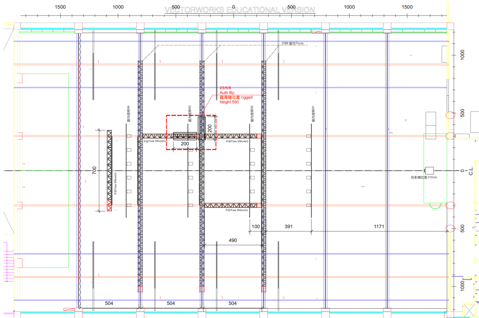
1 FloorPlan Scale: 1:100 Unit: CM
